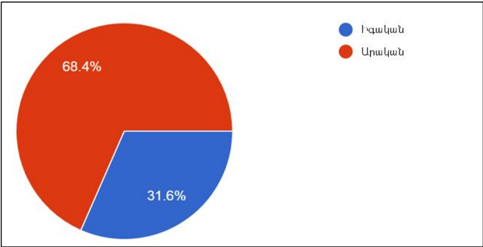
Գծապատկեր 1. Տվյալագետների սեռային բաշխվածությունը ՀՀ-ում
