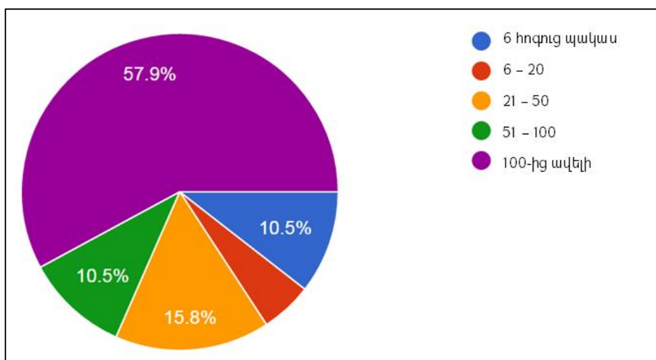
Գծապատկեր 3. Աշխատակիցների քանակը՝ հարցմանը մասնակցած մասնագետների ընկերություններում
