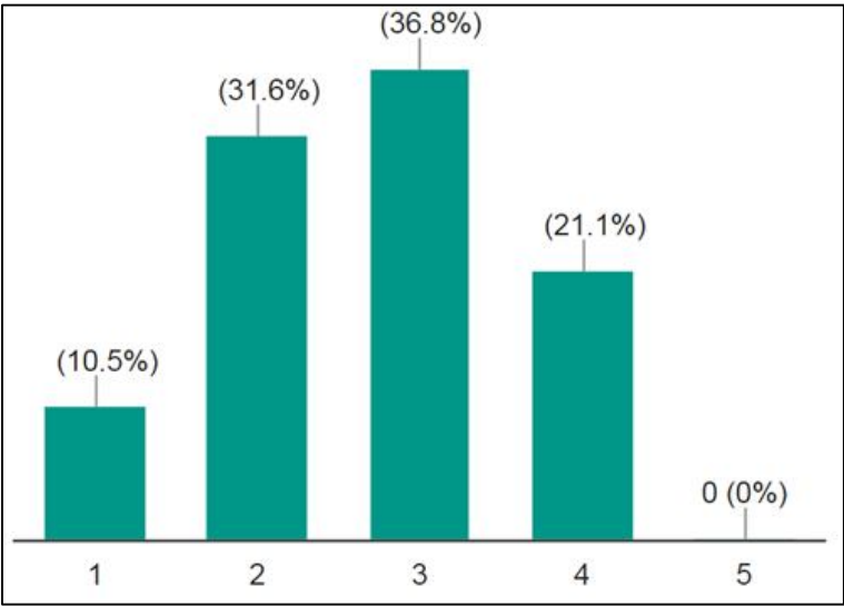
Գծապատկեր 4. Տվյալագետների հմտության սեփական գնահատականը
