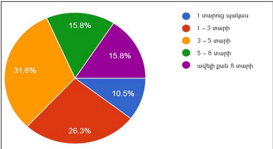
Գծապատկեր 2. Տվյալագետների բաշխվածությունը՝ ըստ մասնագիտական փորձի
